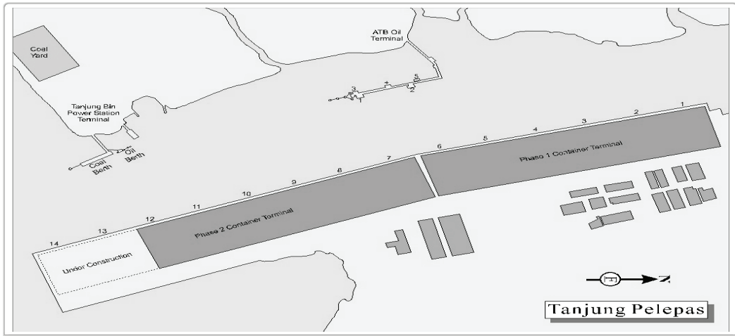
〈그림 IV-9〉 탄중펠레파스항 컨테이너터미널 배치도 2
