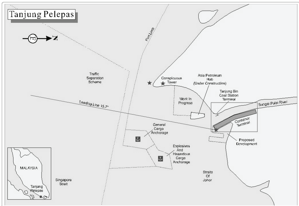
〈그림 IV-8〉 탄중펠레파스항 컨테이너터미널 배치도 1
