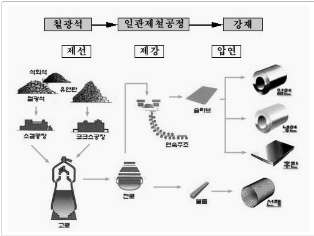
〈그림 Ⅲ-5〉 철강산업의 주요공정
