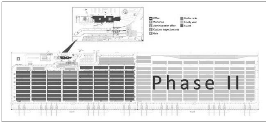
〈그림 IV-8〉 수에즈운하 컨테이너터미널의 레이아웃
