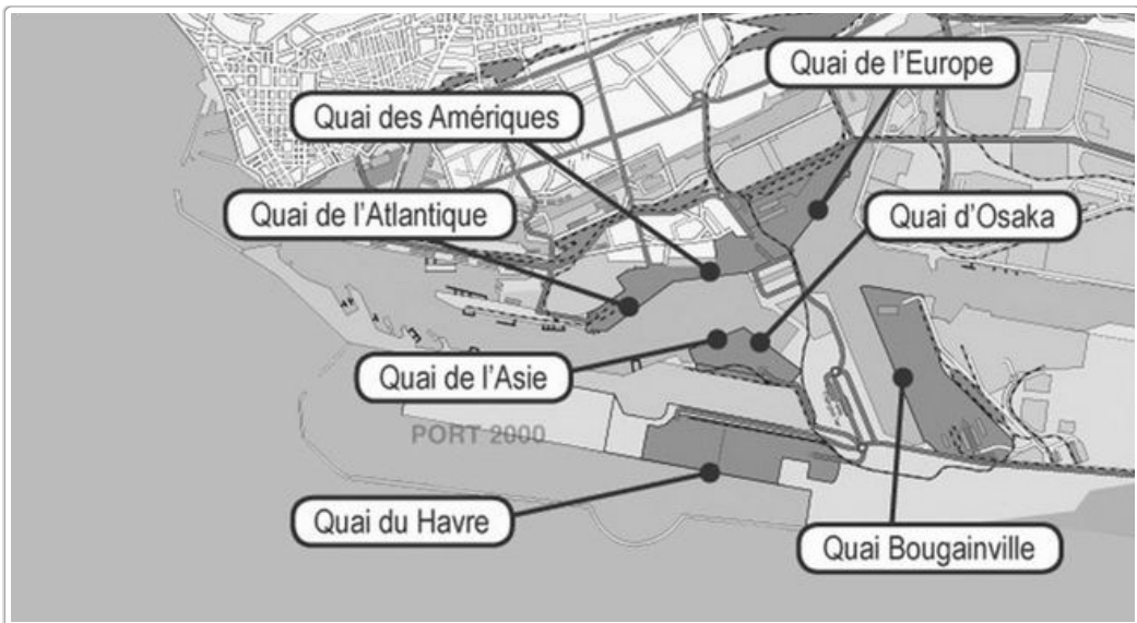
〈그림 IV-12〉 르아브르항 컨테이너터미널 배치도
