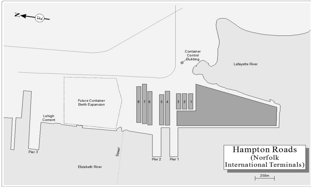
〈그림 IV-4〉 NIT 컨테이너부두 배치도 및 개발 예정도
