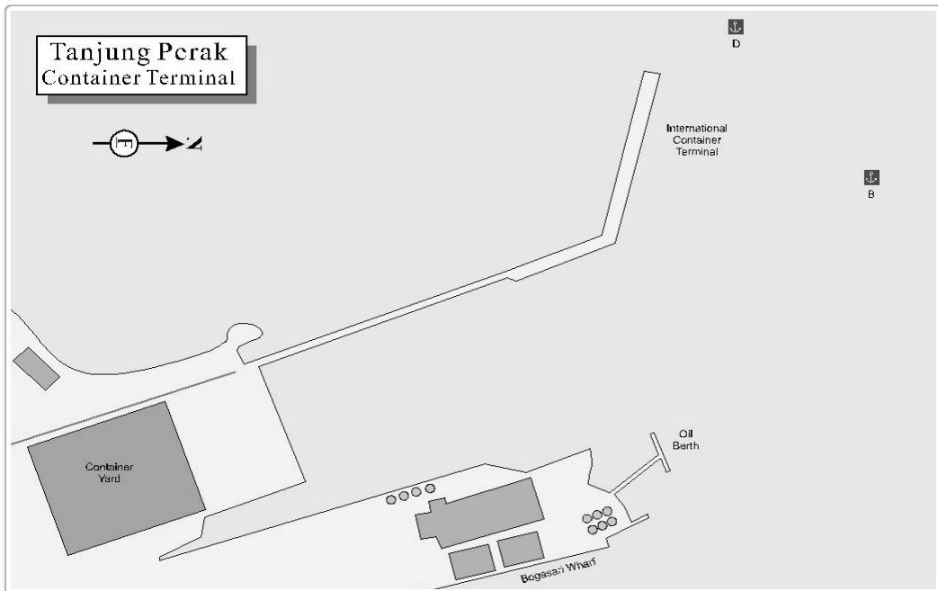
〈그림 IV-10〉 탄중페락항의 컨테이너터미널 배치도
