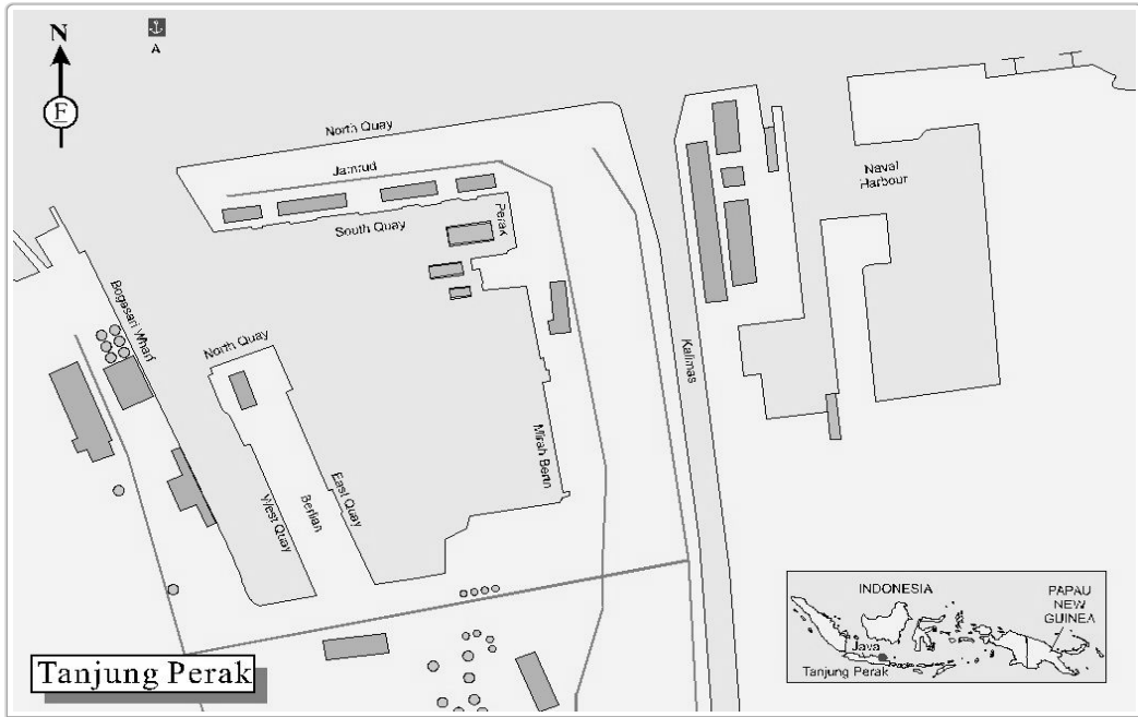
〈그림 IV-9〉 탄중페락항 배치도
