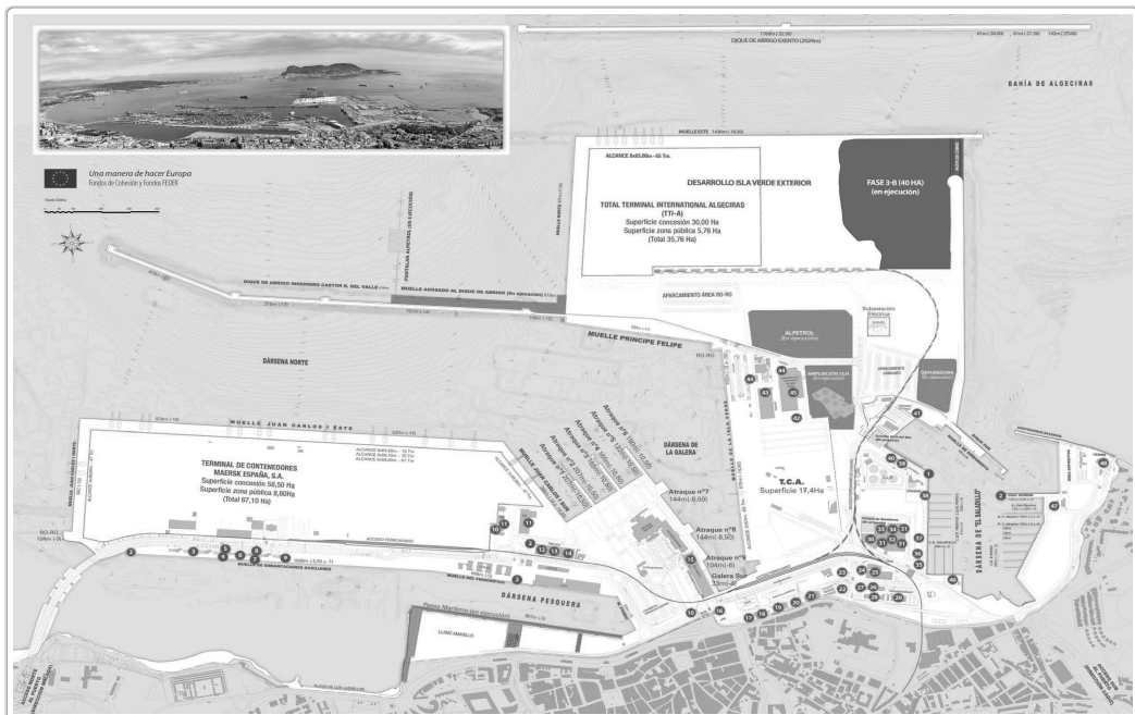
〈그림 IV-14〉 알헤시라스항 배치도(2)
