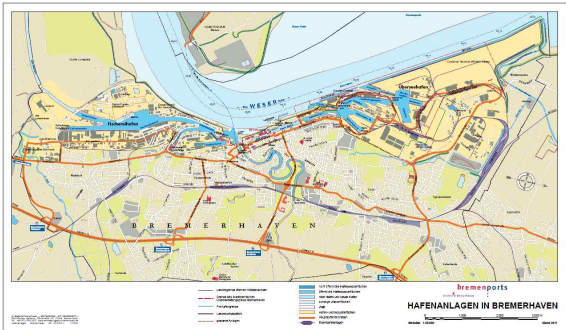
〈그림 IV-6〉 브레머하펜항 배치도
