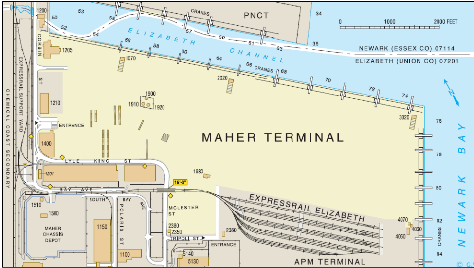
〈그림 IV-7〉 Masher 터미널의 레이아웃
