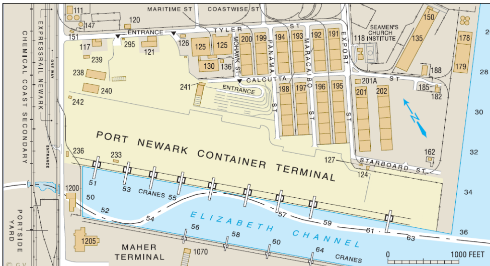
〈그림 IV-8〉 Port Newark 컨테이너터미널의 레이아웃
