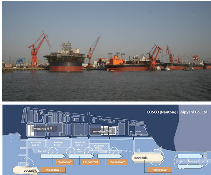
〈그림 III-4〉 Cosco 난통 조선소 전경 및 부두배치도
