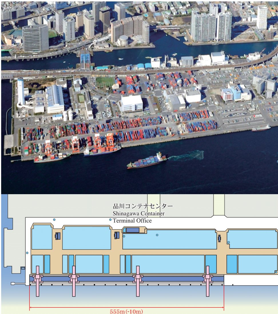
〈그림 IV- 20〉 도쿄항의 시나가와 컨테이너터미널 전경 및 평면도
