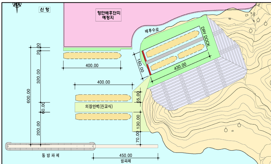
〈그림 III-14〉 부산항 신항 수리조선단지 배치도
