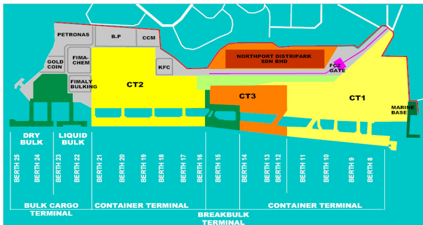
〈그림 IV-13〉 포트클랑항의 North port 터미널 위치 및 부두 배치도
