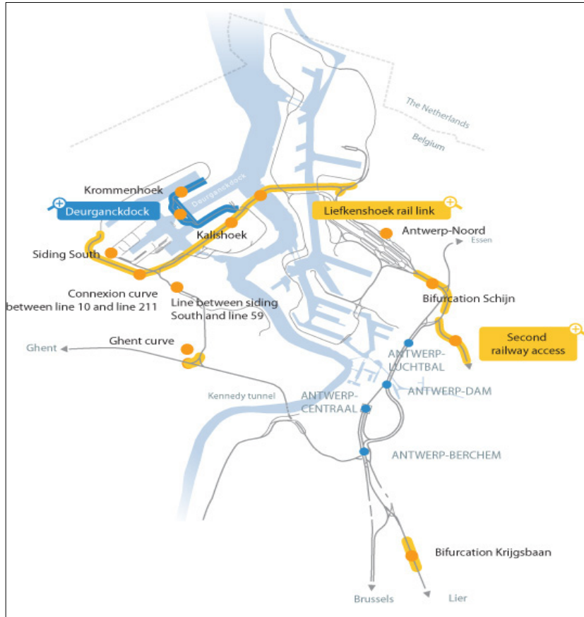
〈그림 IV- 24〉 Deurganck 컨테이너터미널 위치
