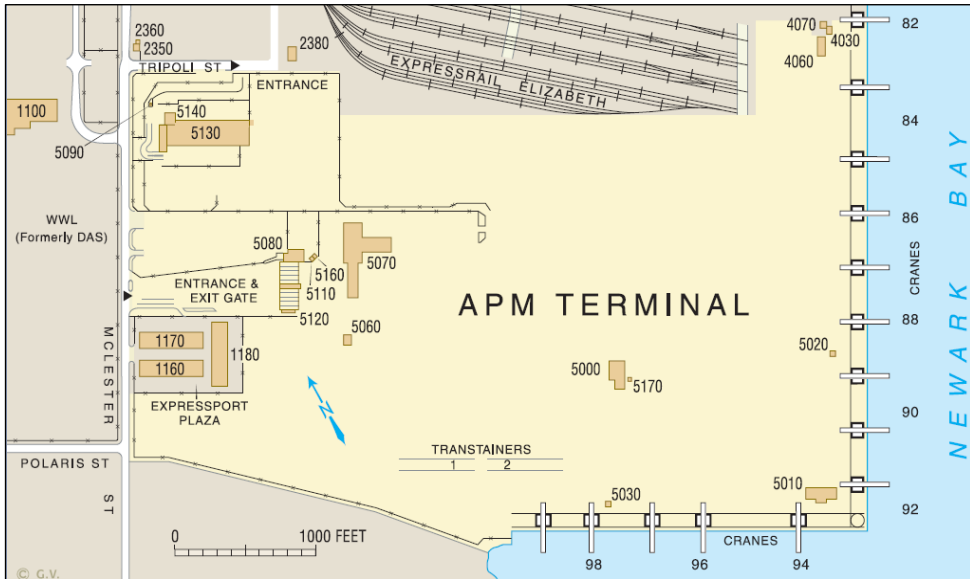
〈그림 IV-5〉 APM 터미널의 레이아웃
