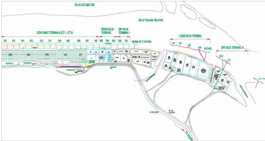
〈그림 IV-14〉 포트클랑항의 West port 터미널 위치 및 부두 배치도
