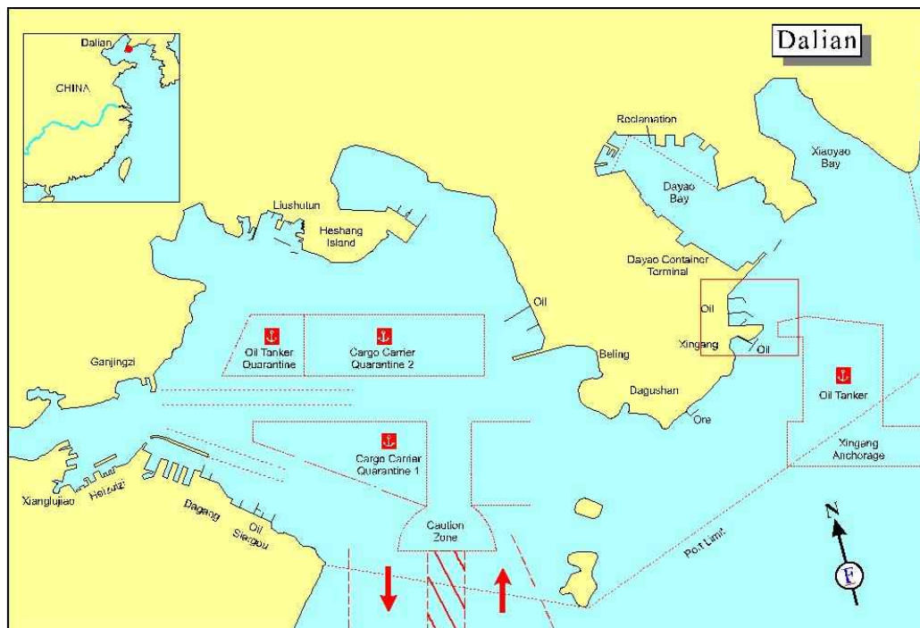
&lt;그림 부록 1-4&gt; 다롄항 시설 현황
