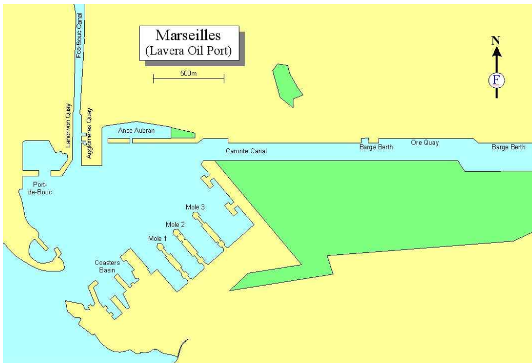
<그림 부록 1-15> 마르세이유항 보조 항만의 배치도(1)
