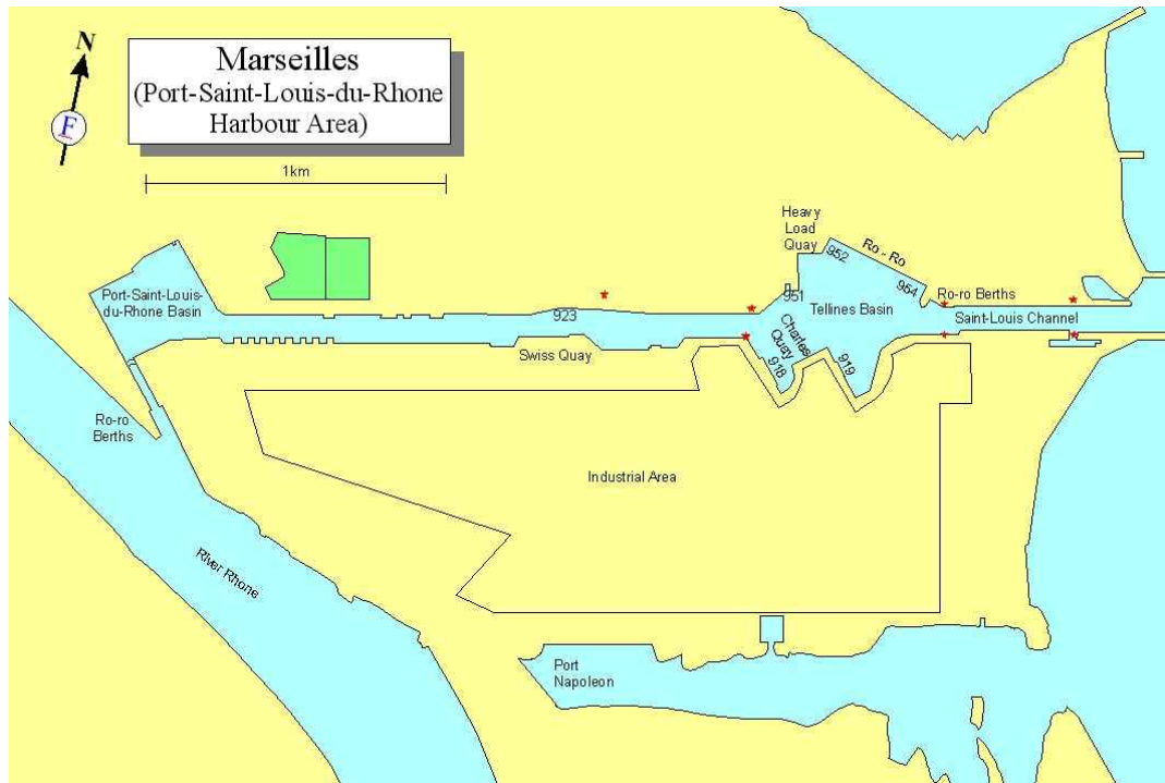
<그림 부록 1-16> 마르세이유항 보조 항만의 배치도(2)
