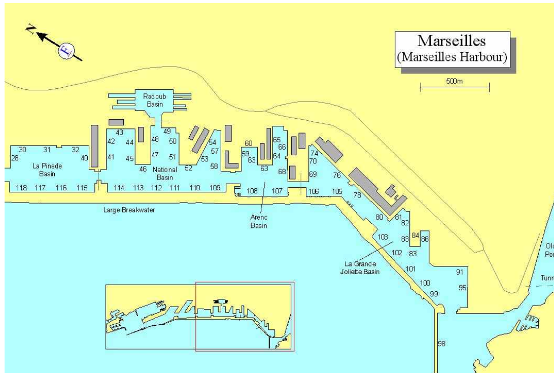
<그림 부록 1-13> 마르세이유항의 부두 배치도(1)
