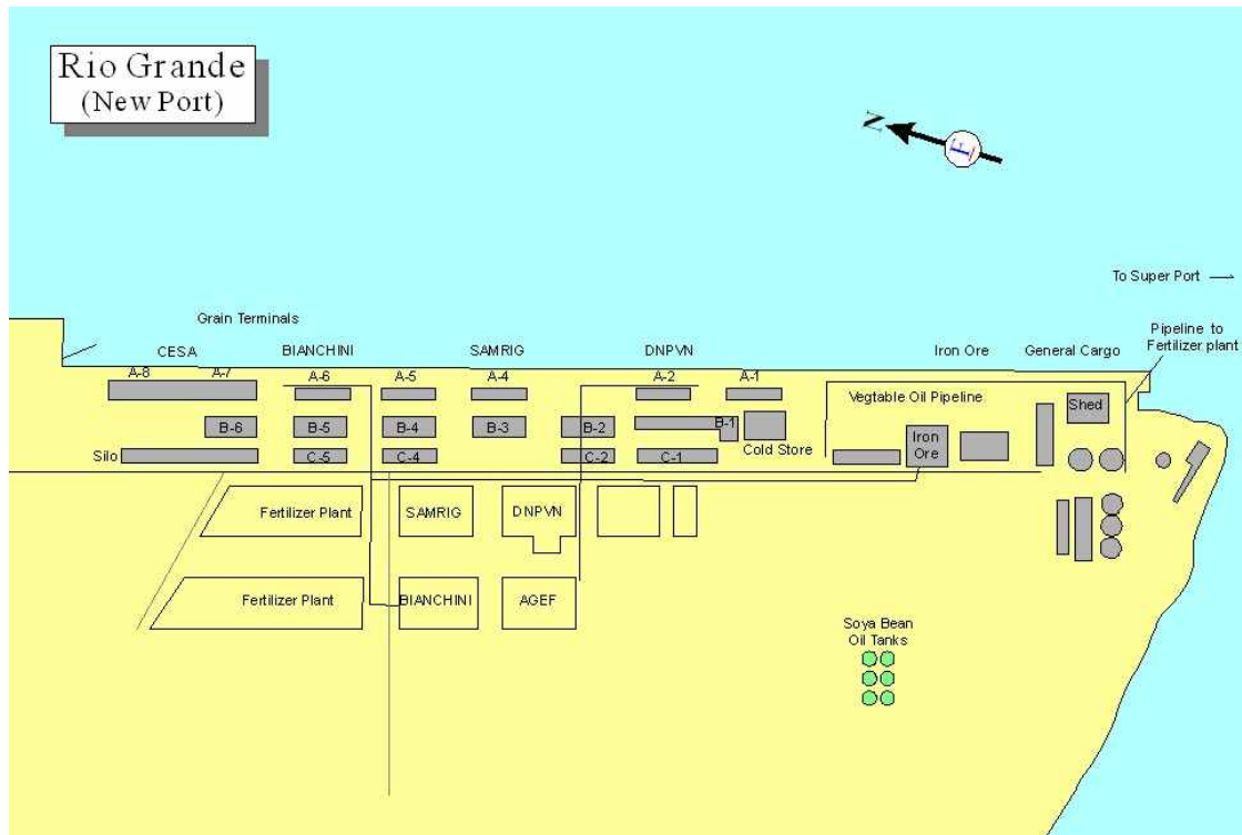
<그림 부록 1-9> 리오그란데항의 부두 배치
