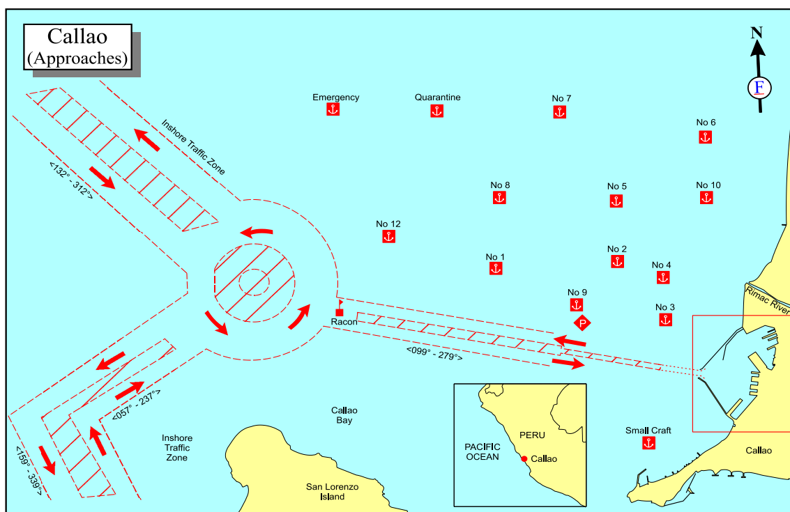
&lt;그림 부록 1-11&gt; 칼라오항 위치와 항내도
