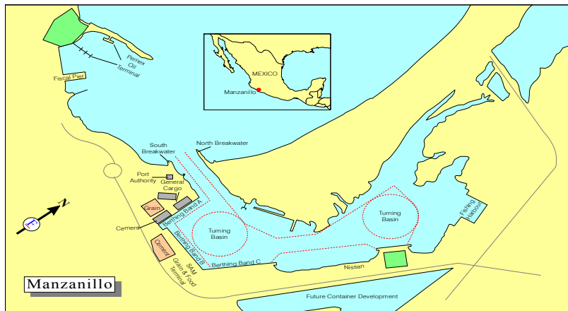
&lt;그림 부록 1-9&gt; 만자닐로항 배치도
