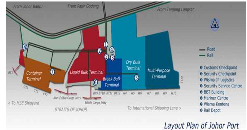
<그림 부록 1-18> 파시르 구당항의 개발 계획 레이아웃
