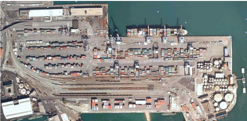
<그림 부록 1-15> Southern European Container Hub Terminal의 배치도
